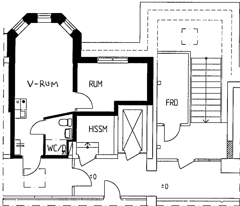
PLAN 6, VINDSVÅNING
